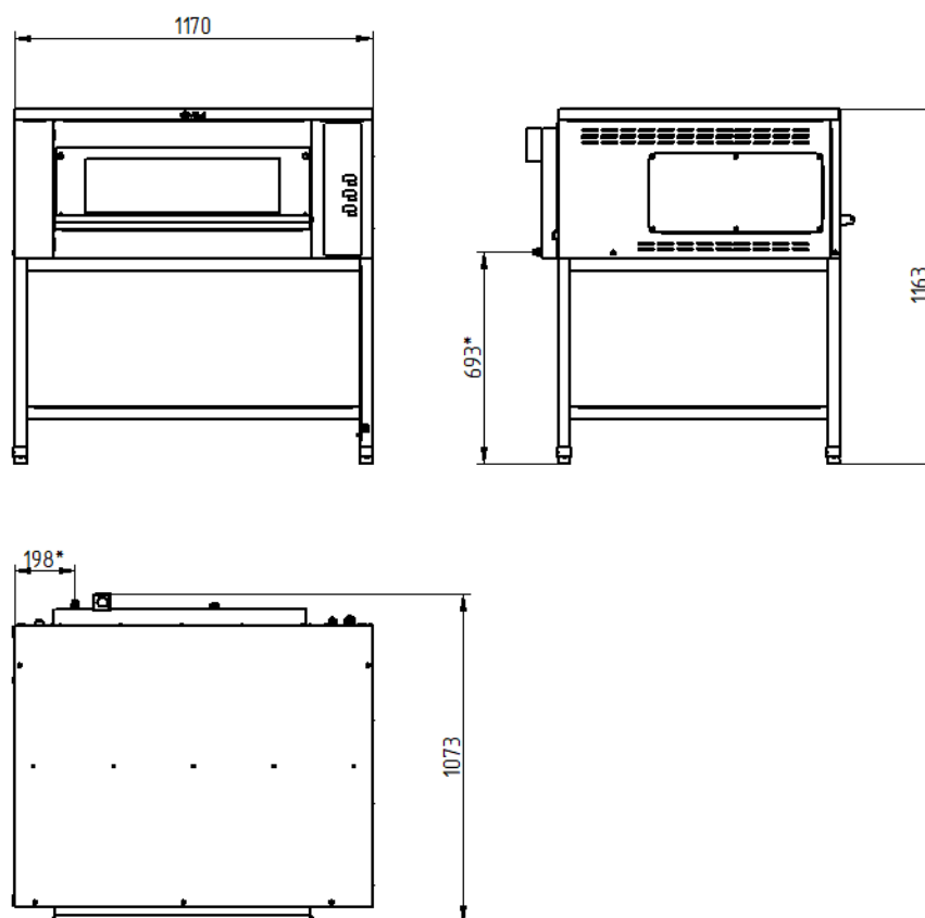
Рис. 2. Общий вид ЭШП-2-01КП 2EN Super.
