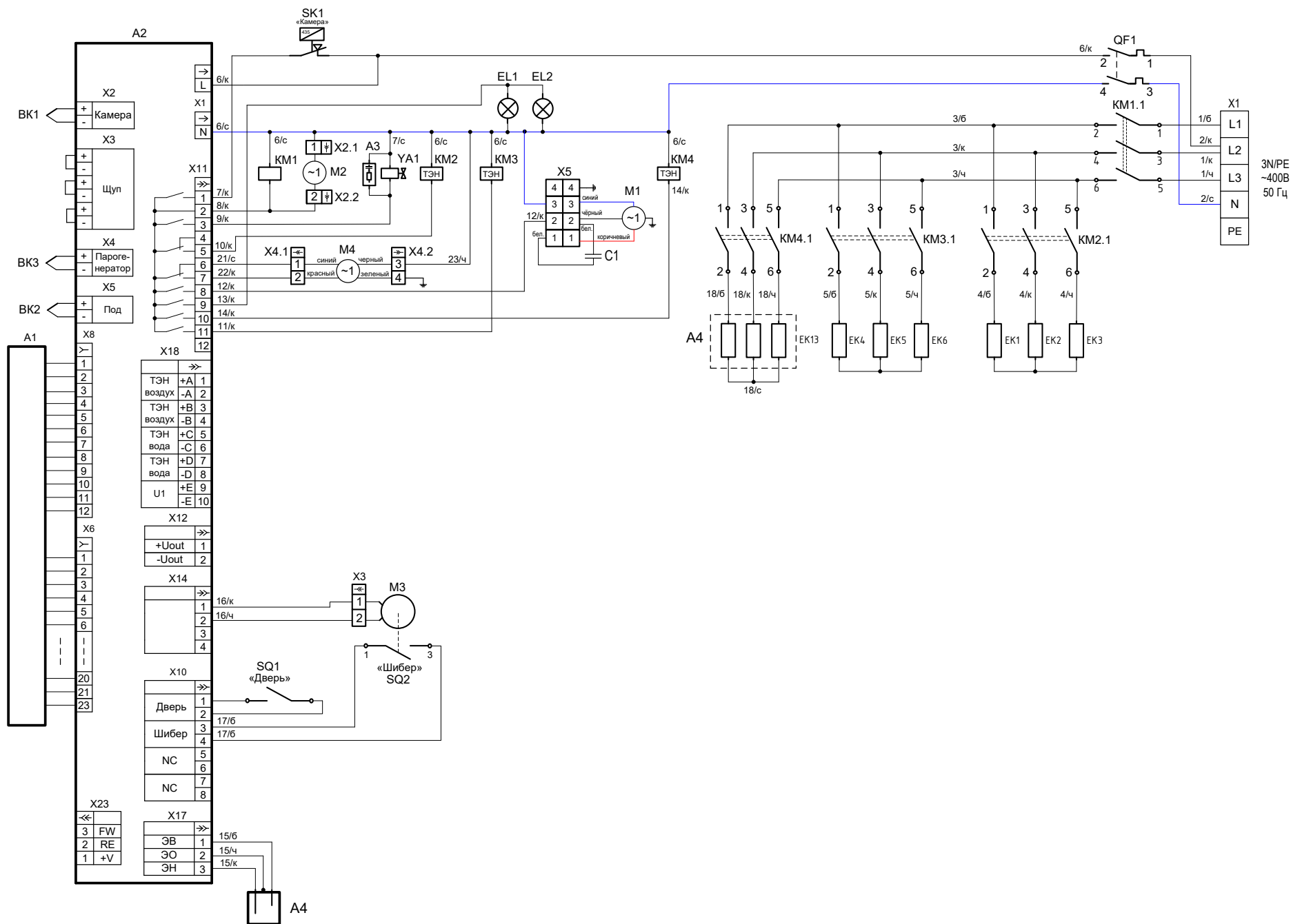
Рис.8 Схема электрическая принципиальная ЭСП-1-01КП 2EN Super с парогенератором
